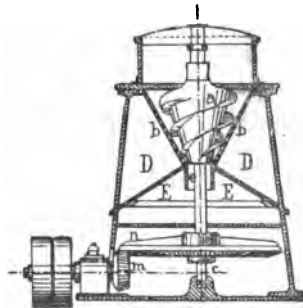
Fig. 63.—Machine à agglomérer Wersmann.
